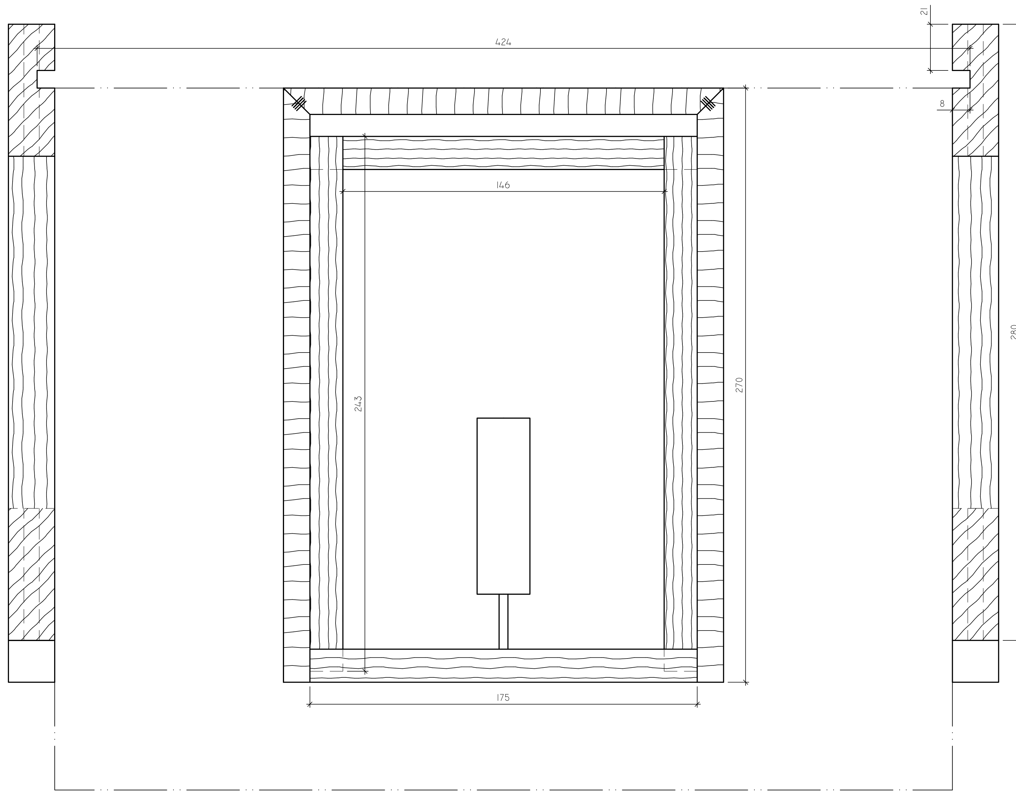
SCHNITT A-A
